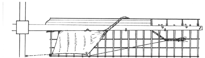
Segel utlagt till höglinan, denna segelyta kallas även högrev.
